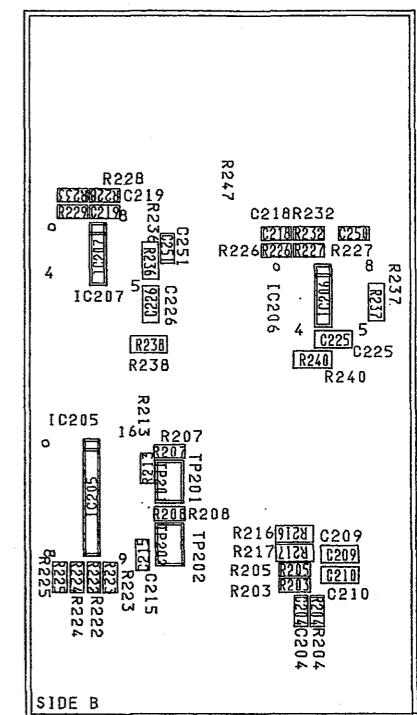
D1 OPTION (PT-1561C) SIDE B
