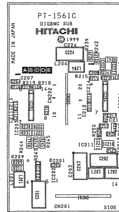
D1 OPTION (PT-1561C) SIDE A
