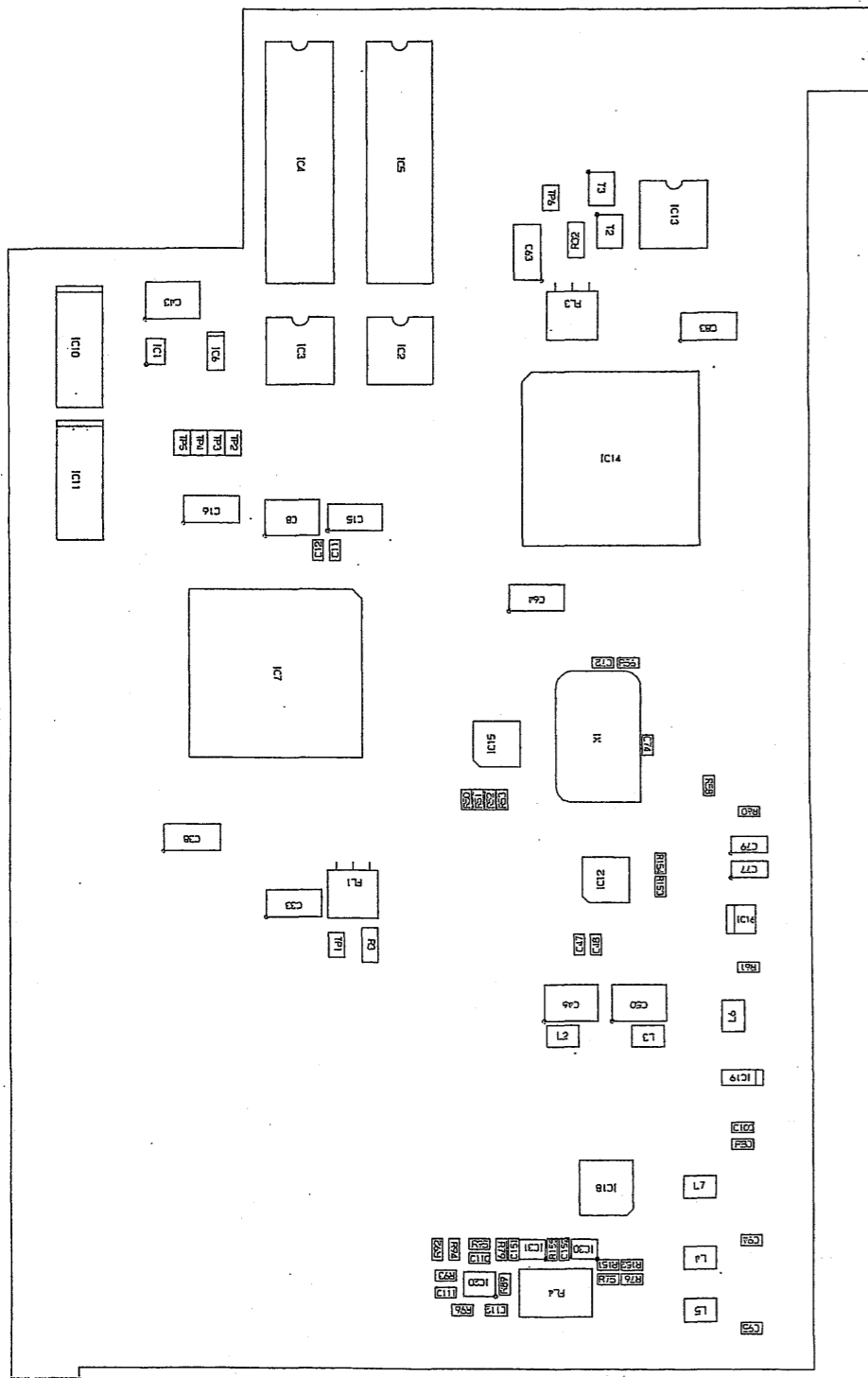
D1 OPTION (PT-1547C) SIDE A
