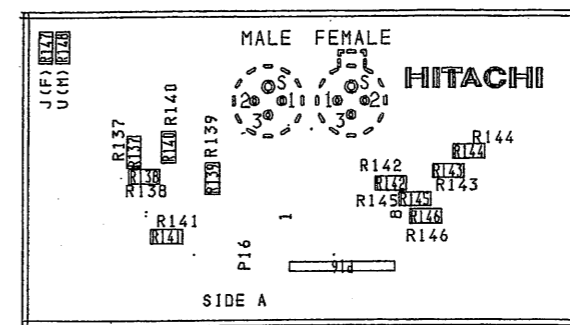
TU-MIC (PT-1543B) SIDE A
