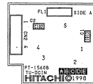
TU-DCIN (PT-1560B) SIDE A
