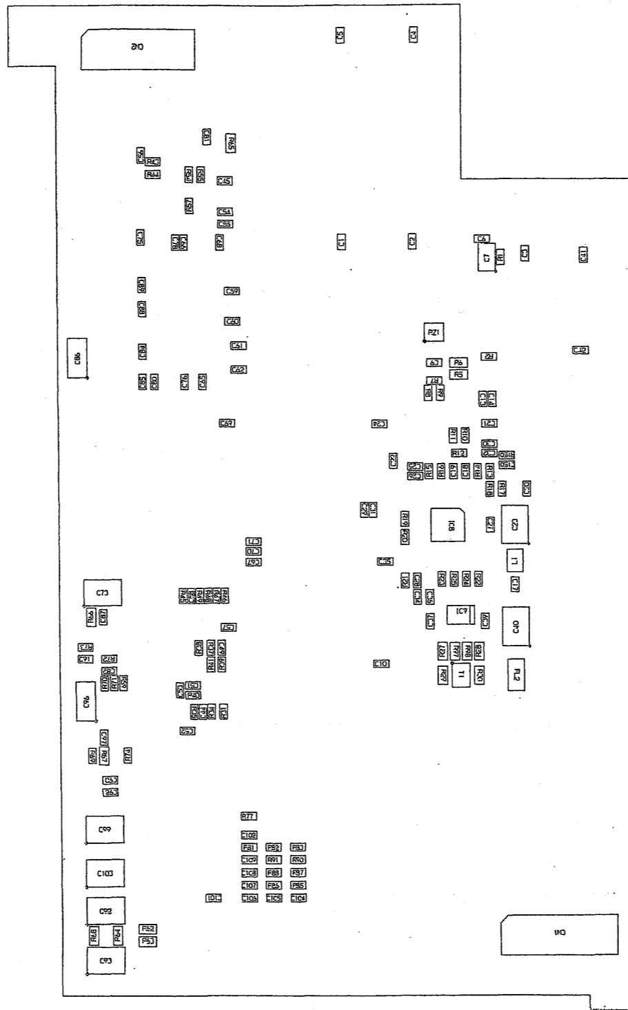
D1 OPTION (PT-1547C) SIDE B
